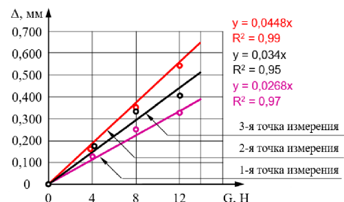
Рисунок 5 – Суммарная деформация модели (рис. 4) в зависимости от точки измерения.
