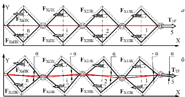
1, 2, i, n – номера тракторных тележек; F_{X1пк} , F_{X2пк} , F_{X1пк} и F_{X2пк} – силы сопротивления качению левых колёс тракторных тележек; F_{X1пк} , F_{X2пк} , F_{X1пк} и F_{X2пк} – силы сопротивления качению правых колёс тракторных тележек; 5 – тракторное водило; T_{TP} – сила тяги трактора.
